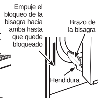
Brazo de la bisagra Bloqueo de la bisagra Extremo inferior de la ranura
