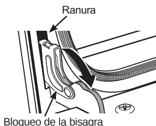
Ranura Bloqueo de la bisagra Empuje los bloqueos de la bisagra hacia abajo para desbloquear
