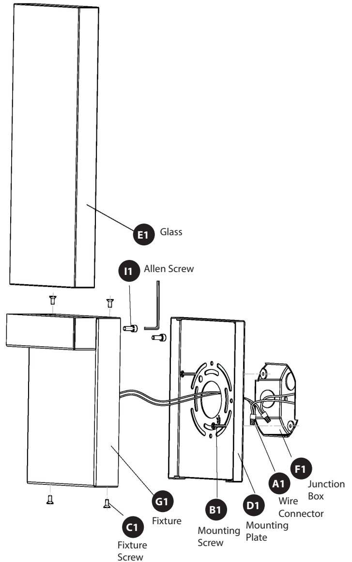
Fig. 2 Wiring
