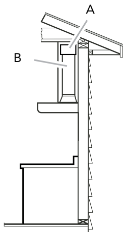
RECIRCULATING MODE
