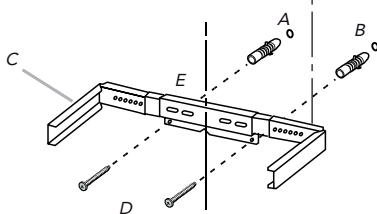
A. Anclajes para tablaroca de 8 x 40 mm B. Línea central en la pared C. Placa de fijación de la cubierta de ventilación
