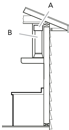
MODE RECIRCULATION
