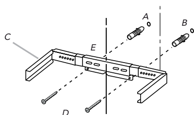
A. Ancrages pour cloison sèche de 8 x 40 mm B. Axe central au mur C. Support de l'abat-vent
