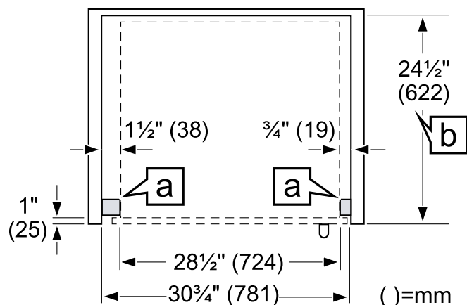
Vue de dessus porte battante droite
