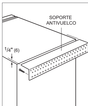
Soporte antivuelco
