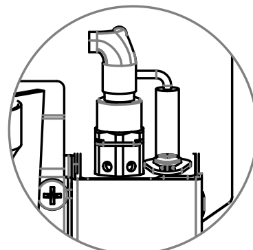
ASSEMBLAGE PILOTE
