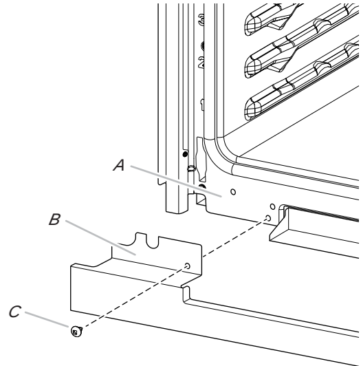
A. Marco del horno B. Lengüeta del protector de la ventilación inferior C. Tornillos n.º 8-18 x 3/8" (9,5 mm)
