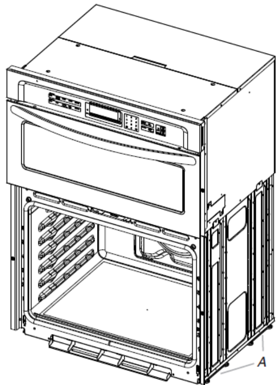
A. Spacers
