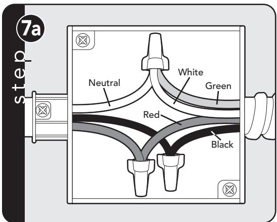
Wiring option 1*
