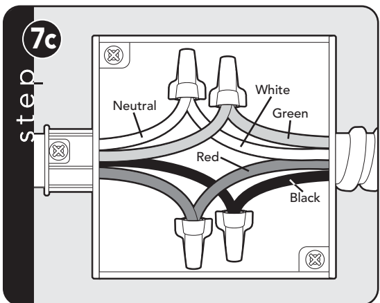
Wiring option 3*
