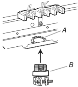
A. Tuerca de retención removible B. Conducto
