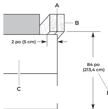
A. Deux panneaux de 2 po x 4 po x 32 po (5 cm x 10 cm x 81 cm) B. Fixer aux montants avec six vis no 8 x 3 po (7,6 cm). C. Couvercle du compresseur D. Distance entre le bas du panneau antibasculement et le plancher
