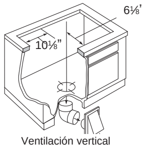
Ventilación vertical
