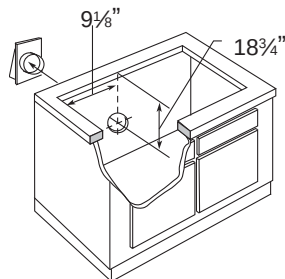
Ventilation par le mur arrière
