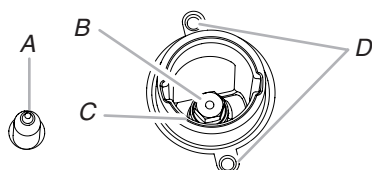
A. Électrode d'allumage B. Injecteur à orifice C. Support d'injecteur à orifice D. Vis
