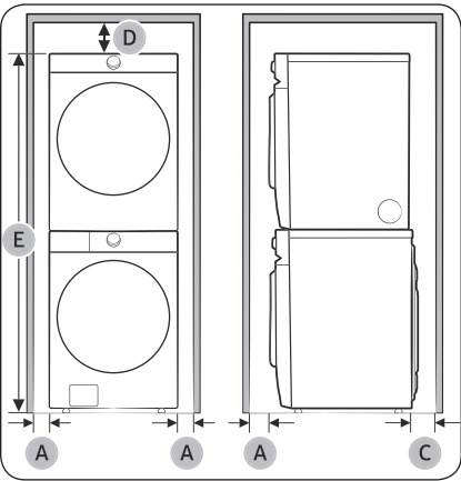
Installation superposée
