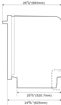
Vue latérale Série DW80R2031
