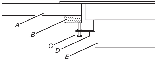
A. Plan de travail B. Cale de bois C. Vis de retenue D. Brides de retenue E. Logement du brûleur
