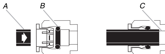
A. Tuyau d'alimentation en eau de ¼" B. Joint torique C. Butée
