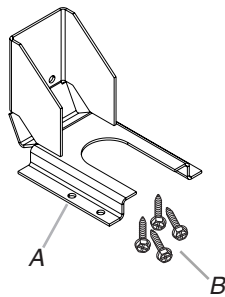
A. Bride antibascullement B. 4 vis à tête Phillips n° 8-18 x 1"
