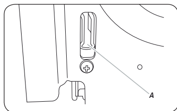
A. Trou à l'intérieur du four pour le verrou de la charnière de la porte
