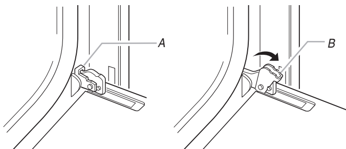
A. Loquet de porte du four en position de verrouillage
