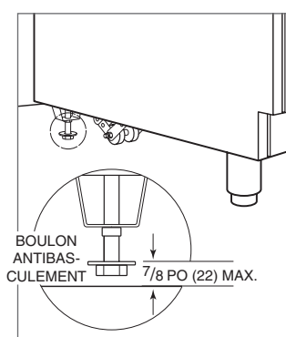
Réglage du boulon antibasculement
