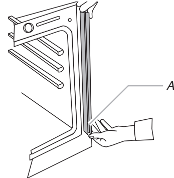
A. Appuyer pour la mise en place de la pièce de garniture et réinstaller la vis.
