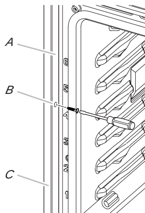
A. Châssis du four B. Trou de la finition latérale C. Finition latérale
