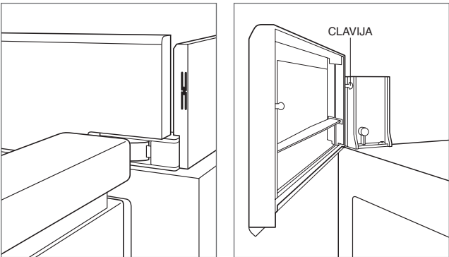
Ribete superior: lado de la bisagra.
