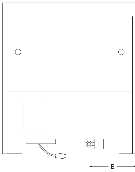
VUE ARRIÈRE
