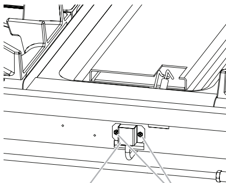
A. Vis B. Support de porte-gicleur de gril
