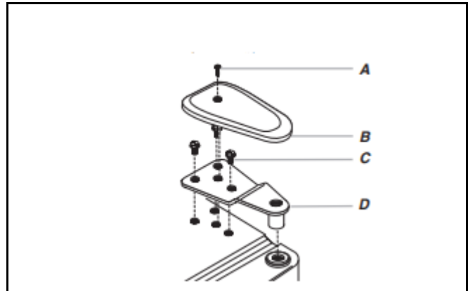
A. Vis du couvre-charnière
